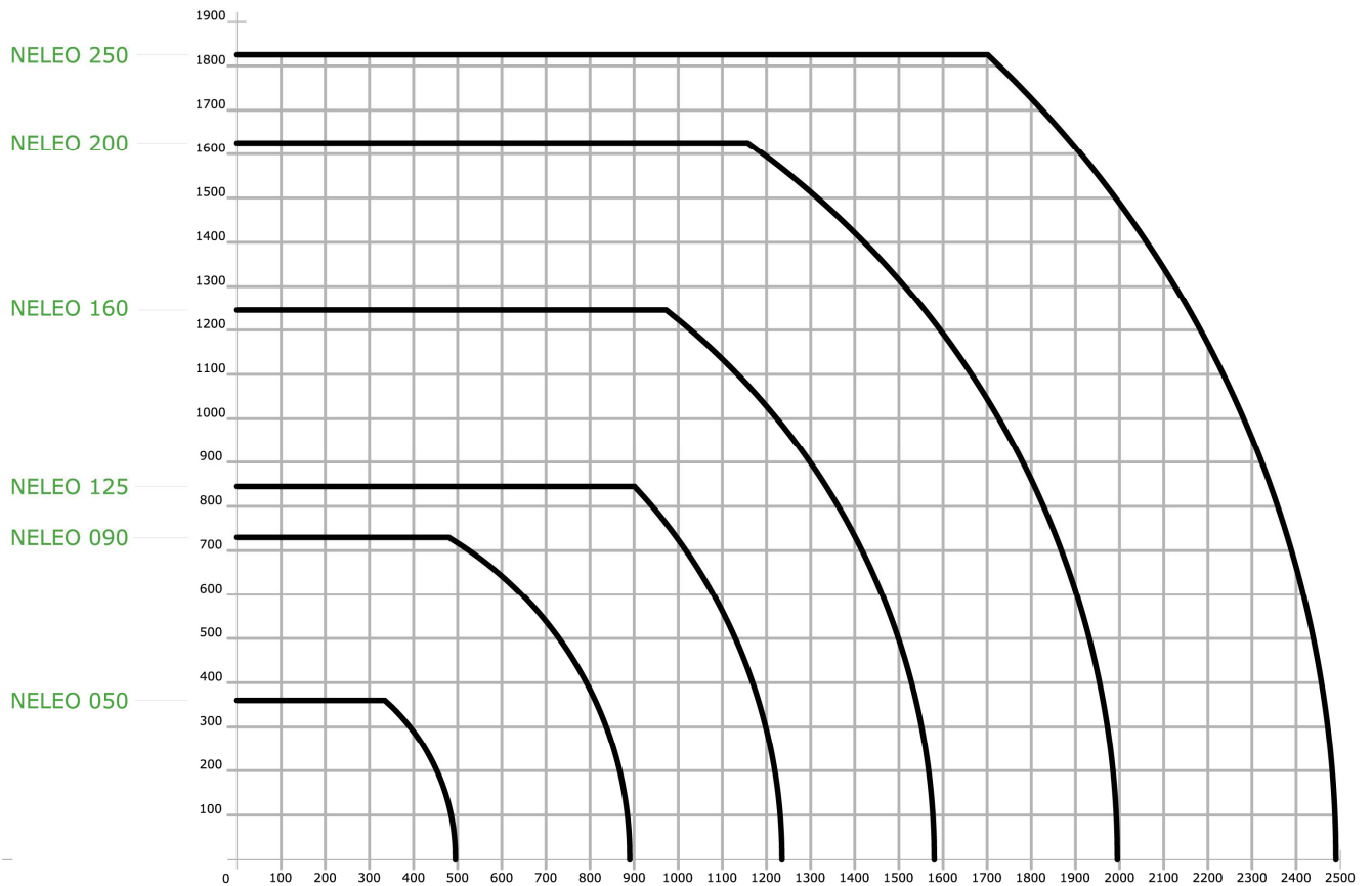
Na rysunku: schemat przeswitu w pierścieniu owijarek NELEO
