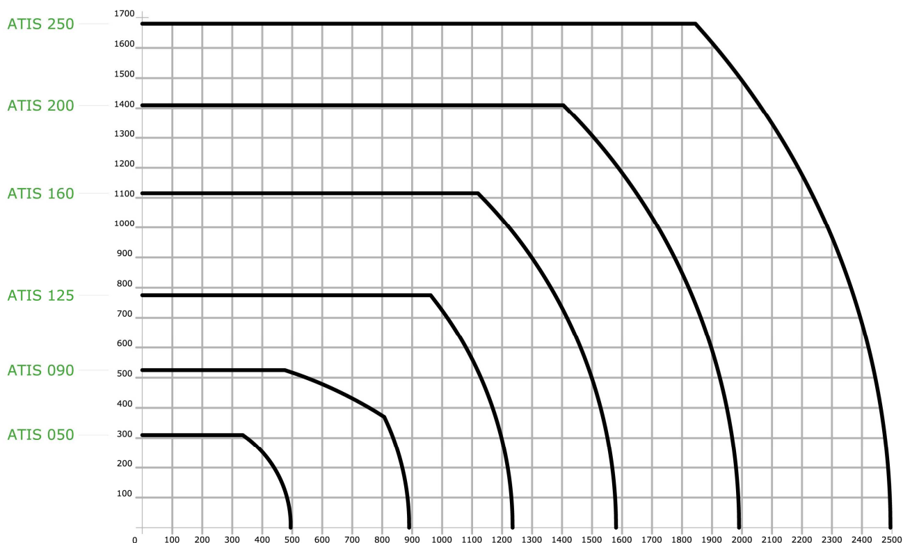
Na rysunku: schemat prześwitu w pierścieniu owijarek ATIS
